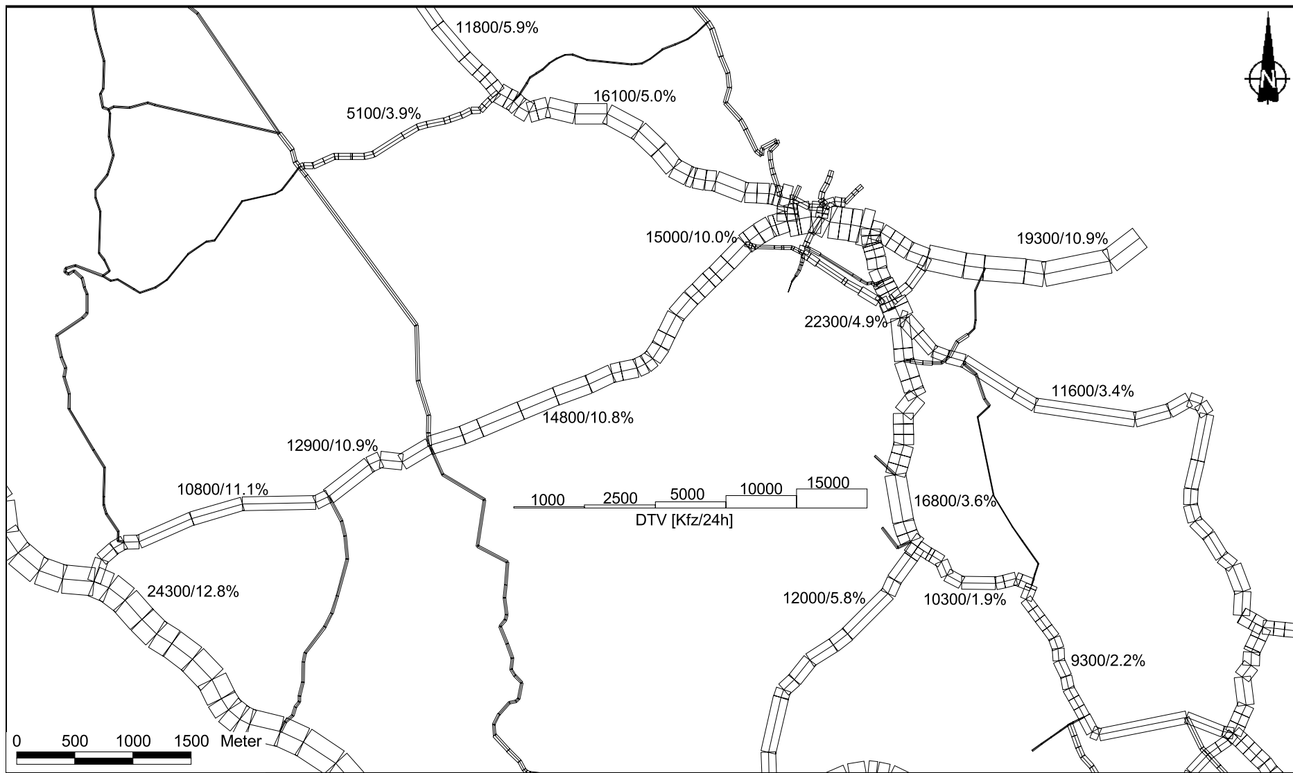
Abb. 4.1: Durchschnittliche tägliche Verkehrsstärke in [Kfz/24h] und LKW-Anteil in [%] auf dem Straßennetz im Untersuchungsgebiet für den Prognosenullfall im Jahr 2025
