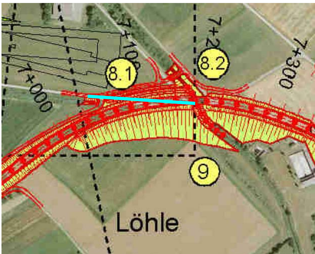
Abb. 3: Ausschnitt aus dem Übersichtsplan zur Trassenlage und Maßnahmenübersicht des LBP für den Bereich der geplanten Lipbachquerung und Teilverlegung. Von der Verlegung betroffener Abschnitt des Lipbachs farblich markiert (hellblau).
